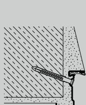
Kutni dovratnik sa skrivenom montažom učvršnicama
