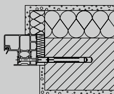
Blok dovratnik Ugradnja u zid od opeke Montaža
