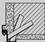
Ugradnja sa zidnim sidrom
