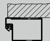
Blok dovratnik za montažu na zid (profil 006) (testirano na suprotnoj strani šarki)
