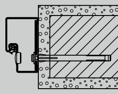
Blok dovratnik Ugradnja u zid od opeke Montaža učvršnicama
