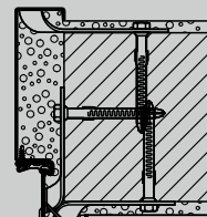
Kutni dovratnik i slijepi dovratnik Ugradnja sa sidrom učvršnice
