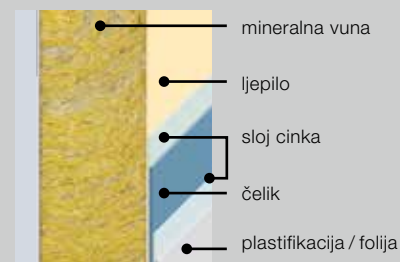
Ispuna od mineralne vune (opcija) za bolju toplinsku izolaciju
