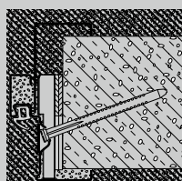
Dijagonalno pričvršćenje s dodatnim okvirom Vario B53 kao sveobuhvatni dovratnik od 2 dijela (porobetun)
