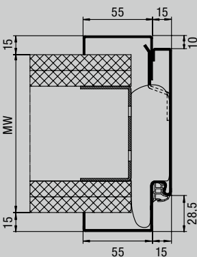
Profil 31103 sa žljebićima
