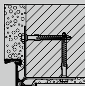
Ugradnja sa sidrom učvršnice
