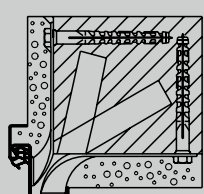
Kutni dovratnik Ugradnja u zid od opeke Sidro za cigleni zid
