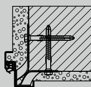
Ugradnja sa sidrom učvršnice
