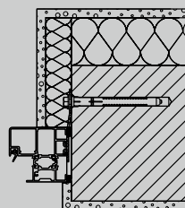
Blok dovratnik Montaža sidrom
