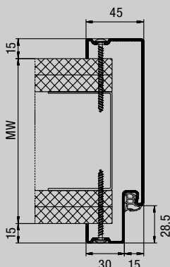
Profil 21120 Zrcalno pričvršćenje vijcima
