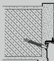
Kutni dovratnik i slijepi dovratnik sa skrivenom montažom učvršnicama
