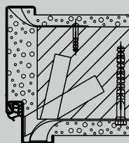
Sveobuhvatni dovratnik Ugradnja u zid od opeke Sidro za cigleni zid
