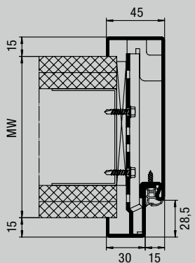
Profil 21180 sa žljebićima
