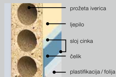
Iverica prožeta cjevastim otvorima (standard)
